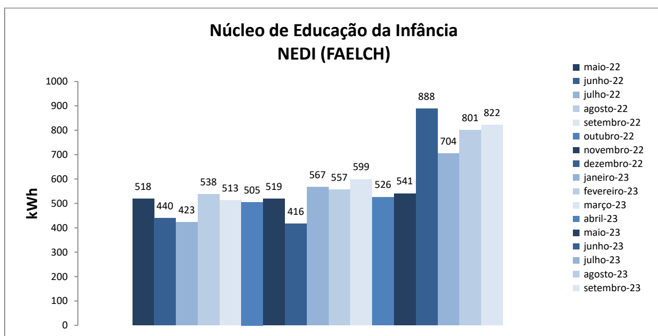
Figura 1. Variação do consumo de energia elétrica da edificação do Núcleo de Educação da Infância - NEDI.
