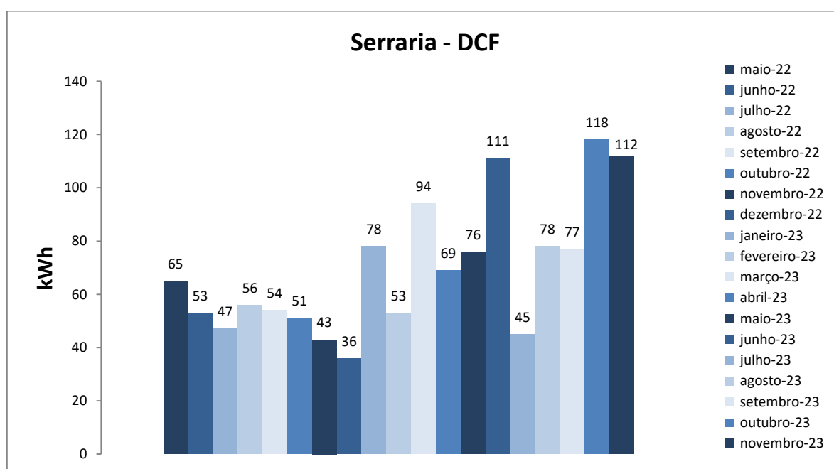
Figura 1. Variação do consumo de energia elétrica da edificação Serraria.
