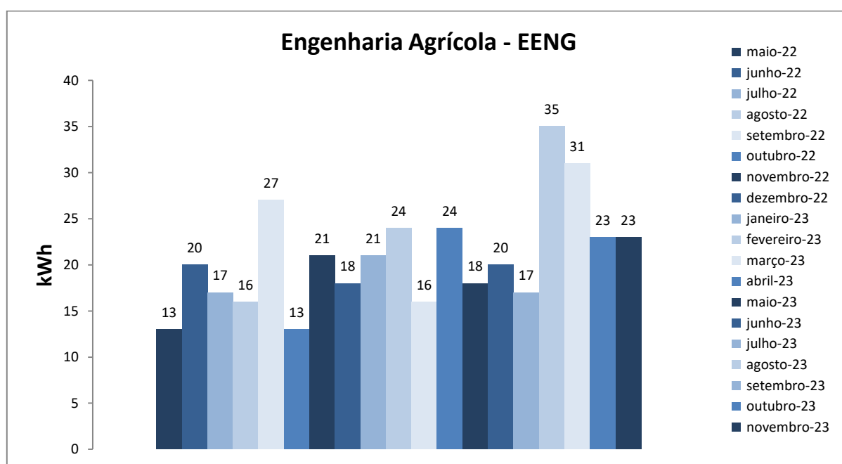
Figura 1. Variação do consumo de energia elétrica da edificação da Engenharia Agrícola.
