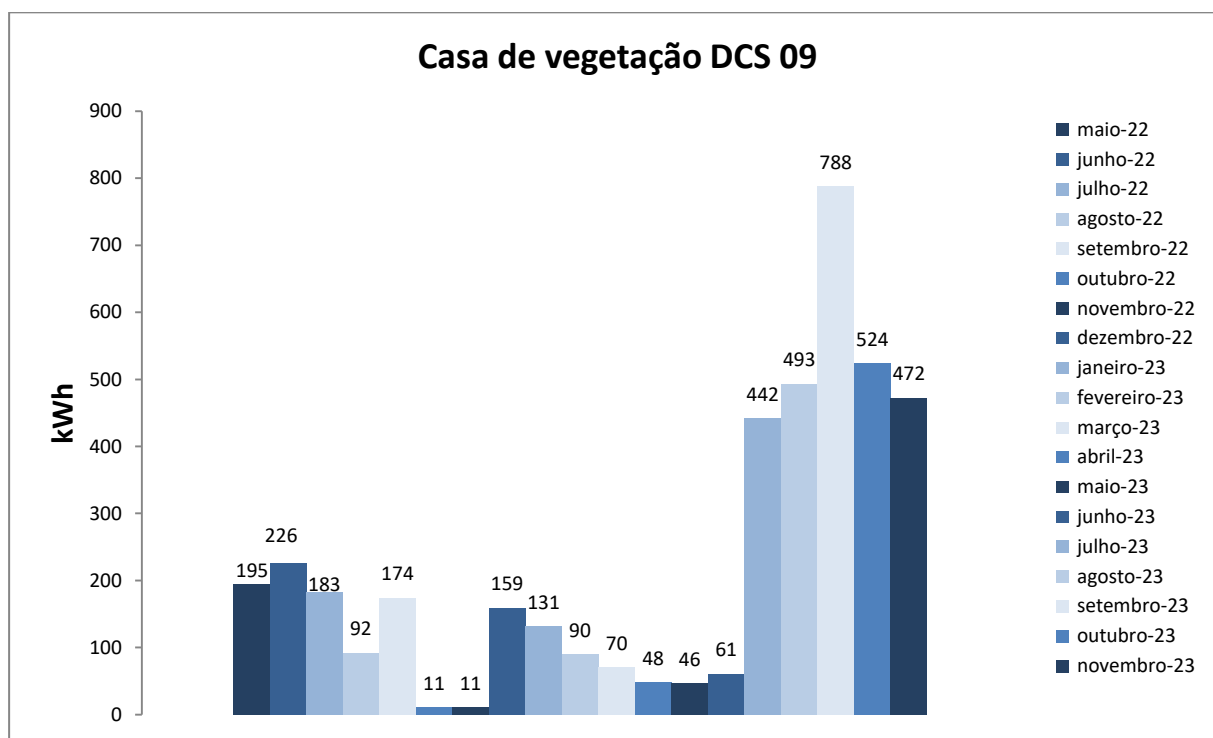
Figura 1. Variação do consumo de energia elétrica da edificação do Departamento de Ciência do Solo Casa de Vegetação 09
