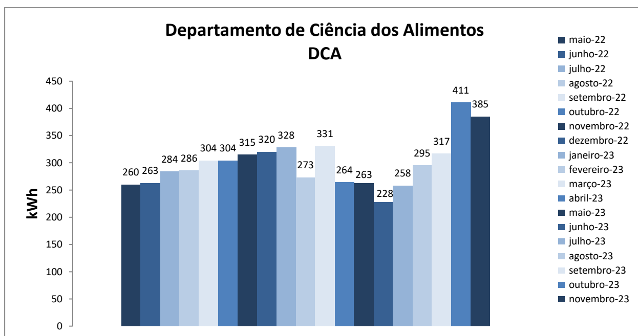
Figura 1. Variação do consumo de energia elétrica das edificações do Departamento de Ciência dos Alimentos.
