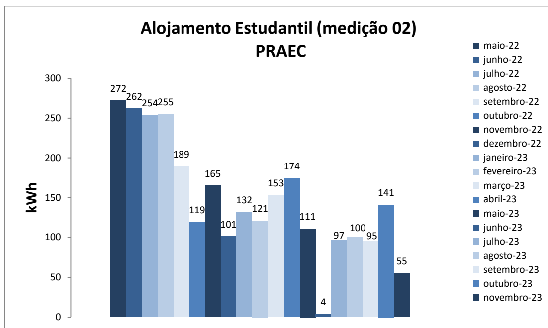
Figura 1. Variação do consumo de energia elétrica da edificação do Alojamento Estudantil – medição 02.
