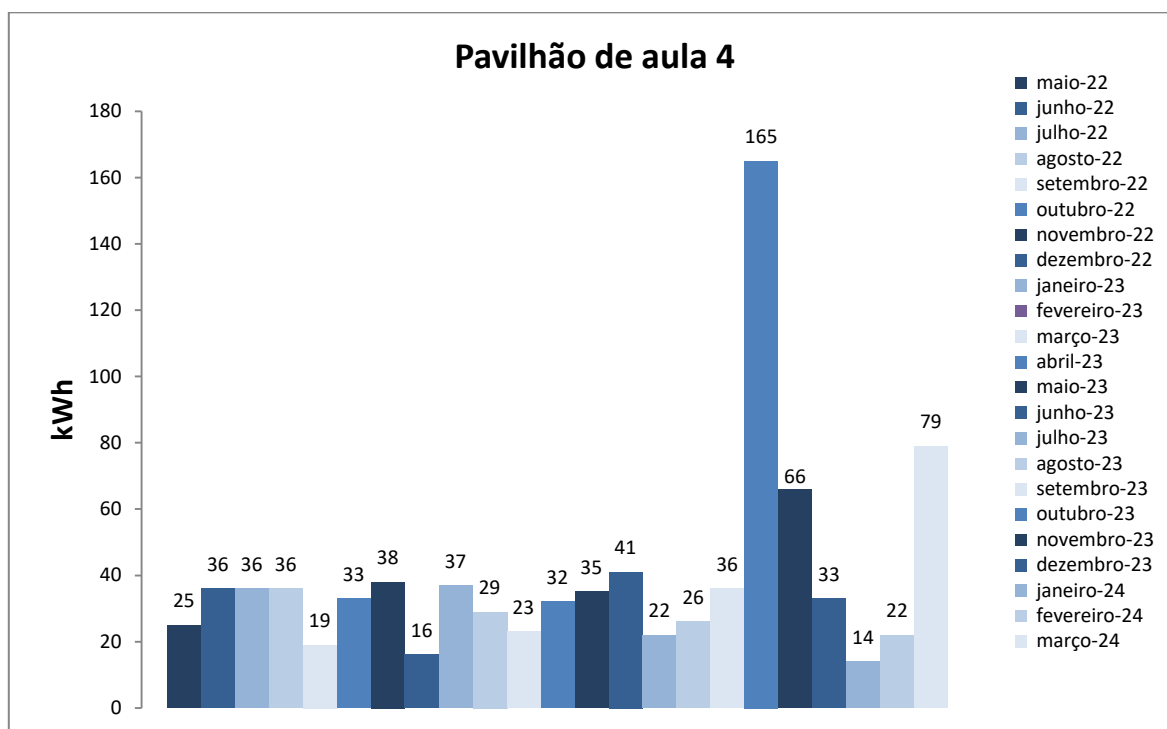
Figura 1. Variação do consumo de energia elétrica da edificação do Pavilhão de Aulas 04.
