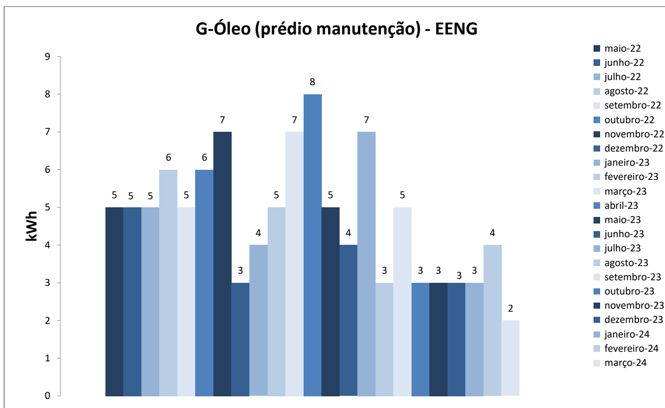
Figura 1. Variação do consumo de energia elétrica da edificação G-Óleo prédio manutenção.
