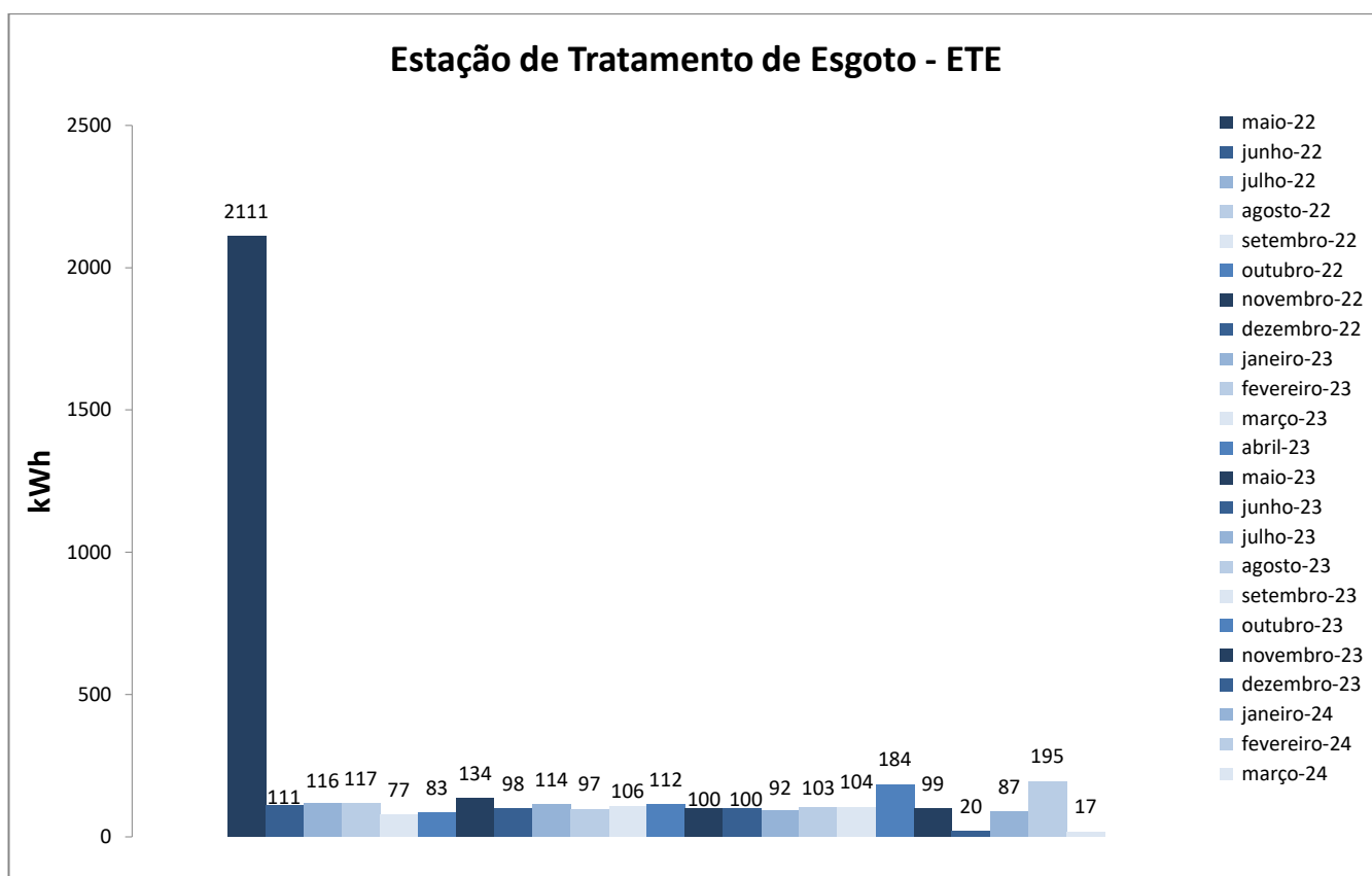
Figura 1. Variação do consumo de energia elétrica da Estação de Tratamento de Esgoto – ETE.
