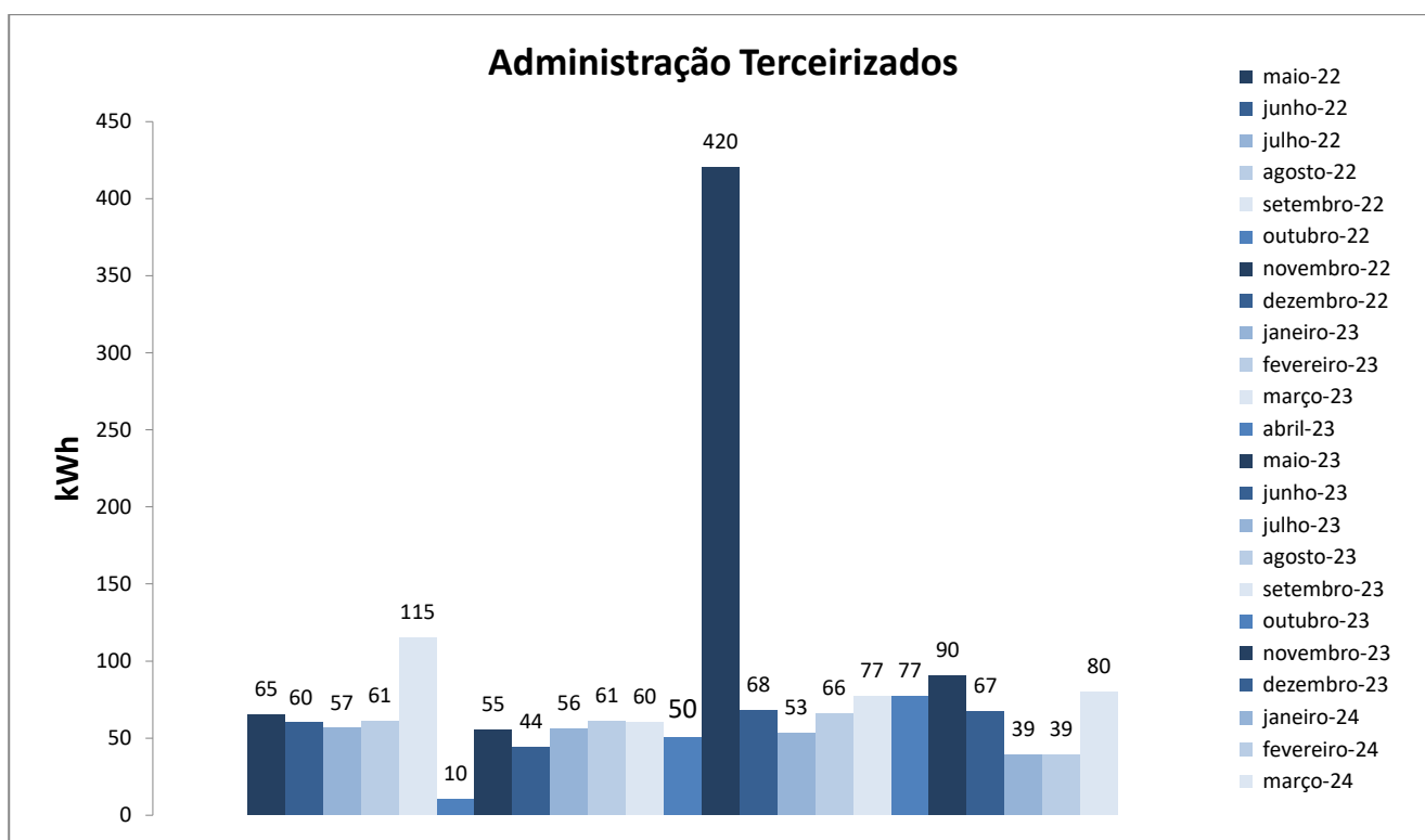
Figura 1. Variação do consumo de energia elétrica do prédio Administrativo Empresas Terceirizadas
