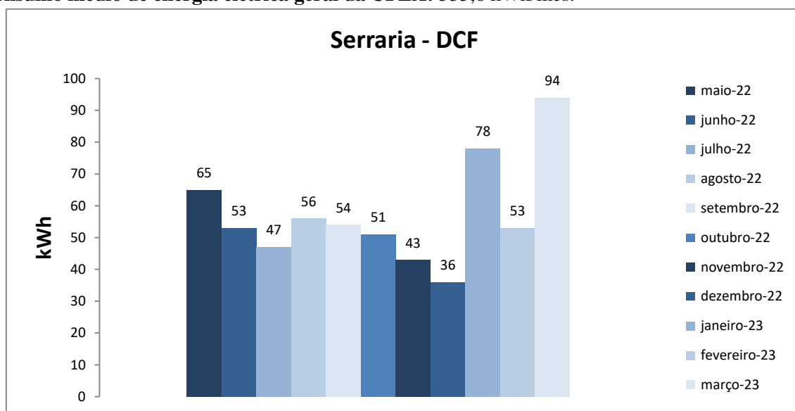
Figura 1. Variação do consumo de energia elétrica da edificação Serraria.
