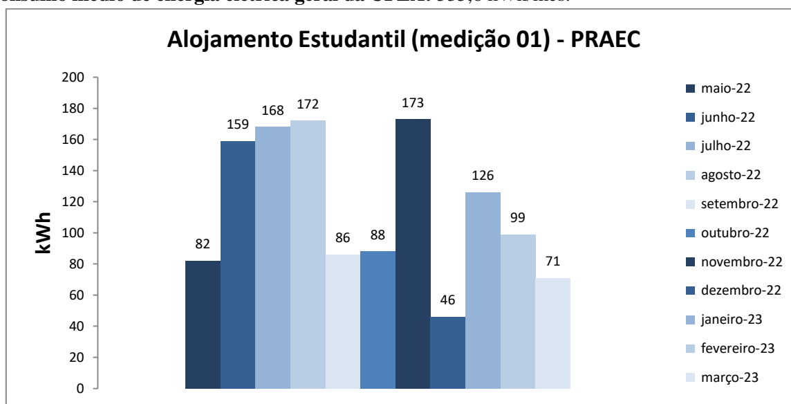
Figura 1. Variação do consumo de energia elétrica da edificação do Alojamento Estudantil – medição 01
