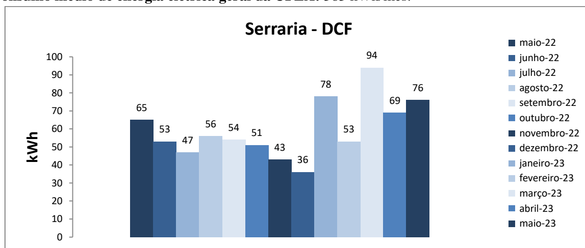
Figura 1. Variação do consumo de energia elétrica da edificação Serraria.
