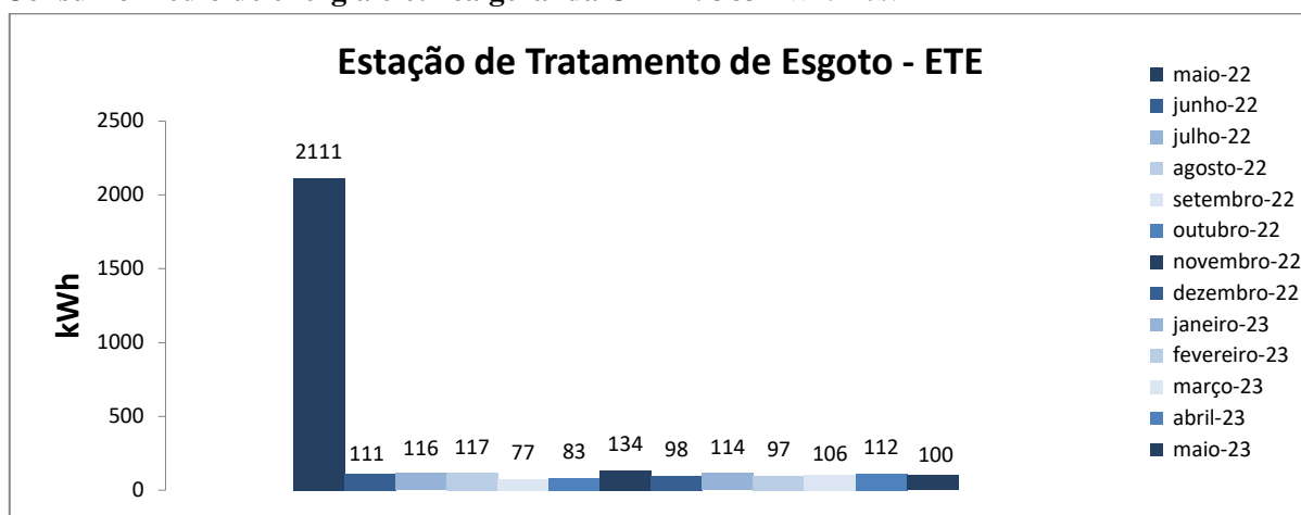
Figura 1. Variação do consumo de energia elétrica da Estação de Tratamento de Esgoto – ETE.
