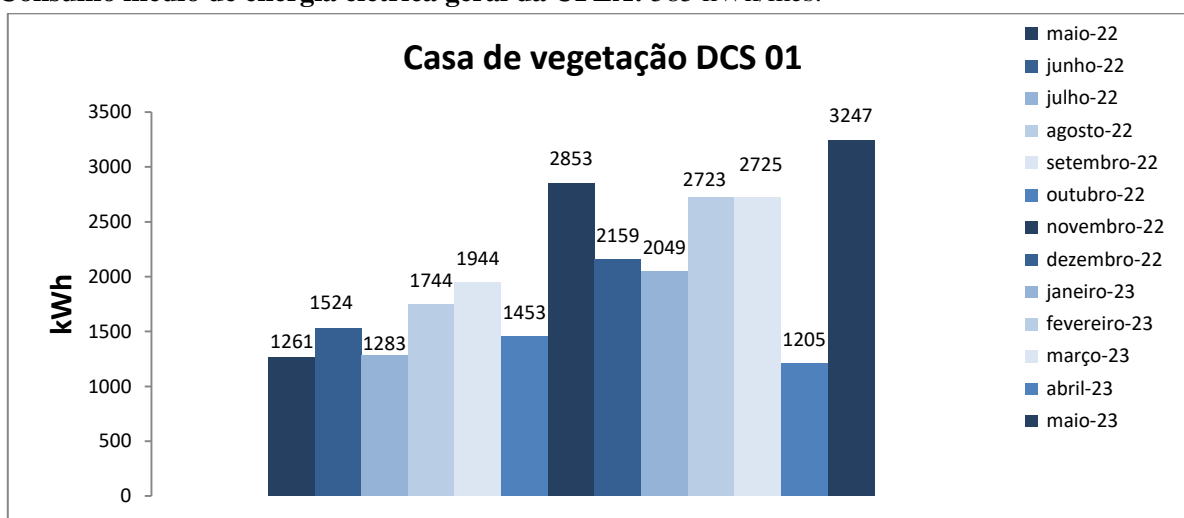
Figura 1. Variação do consumo de energia elétrica da edificação do Departamento de Ciência do Solo Casa de Vegetação 01
