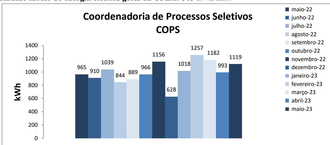
Figura 1. Variação do consumo de energia elétrica da edificação da Coordenadoria de Processos Seletivos
