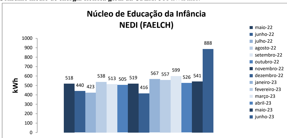
Figura 1. Variação do consumo de energia elétrica da edificação do Núcleo de Educação da Infância - NEDI.
