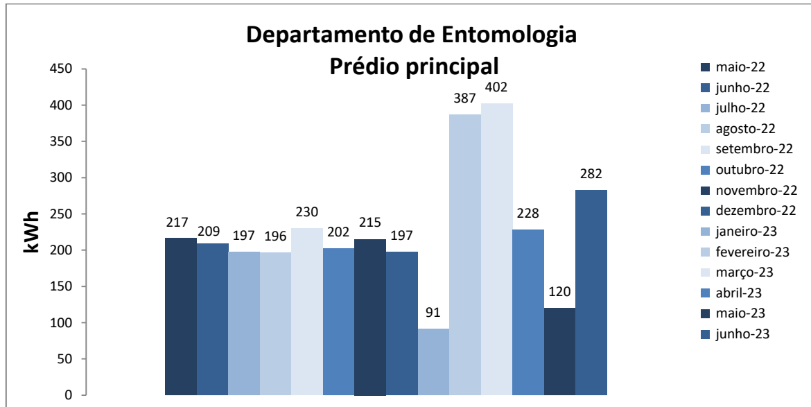
Figura 1. Variação do consumo de energia elétrica da edificação do Departamento de Entomologia
