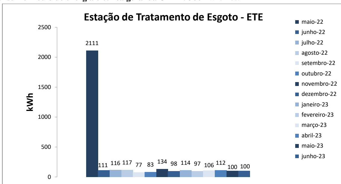
Figura 1. Variação do consumo de energia elétrica da Estação de Tratamento de Esgoto – ETE.
