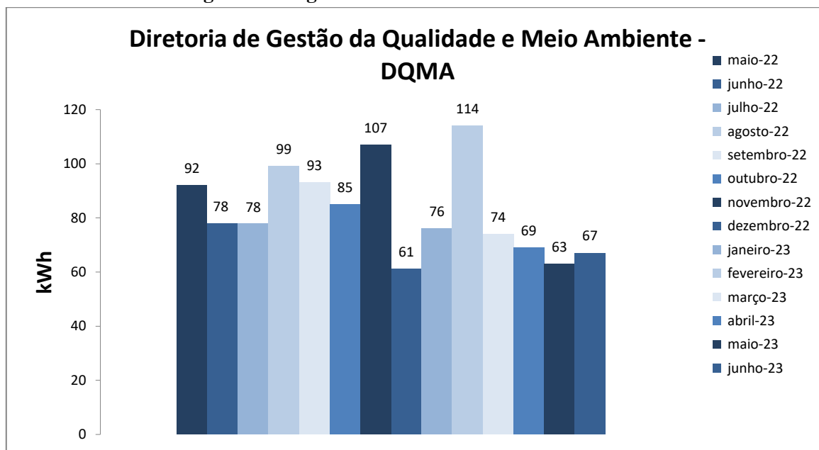
Figura 1. Variação do consumo de energia elétrica do prédio da DQMA
