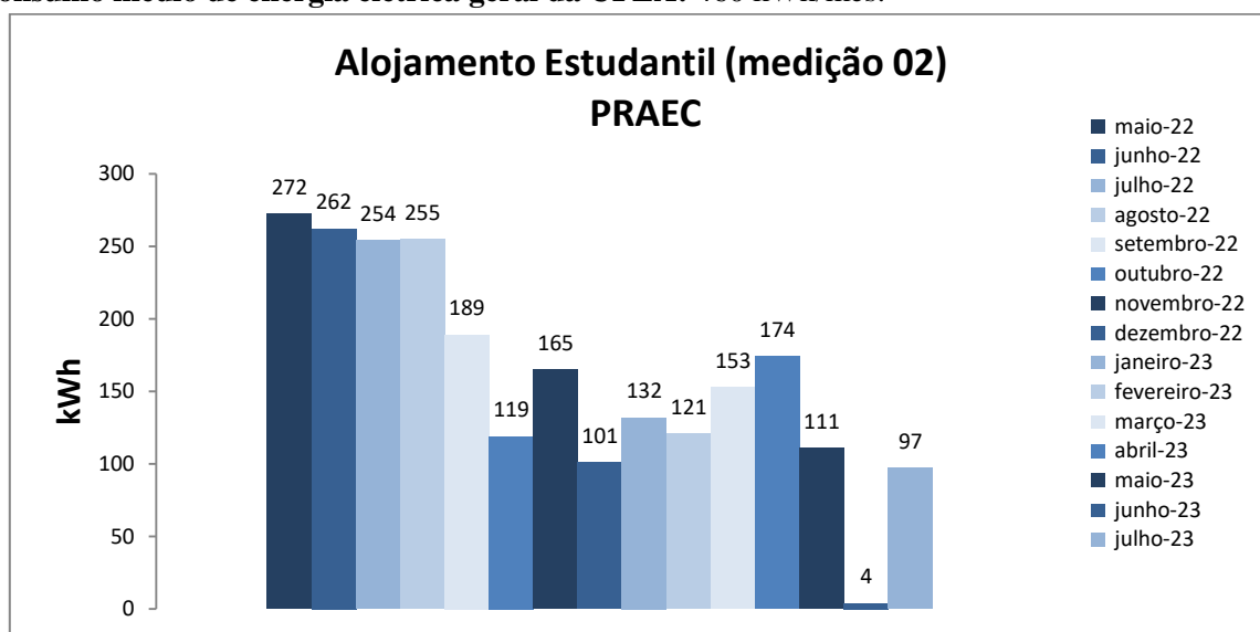
Figura 1. Variação do consumo de energia elétrica da edificação do Alojamento Estudantil – medição 02.
