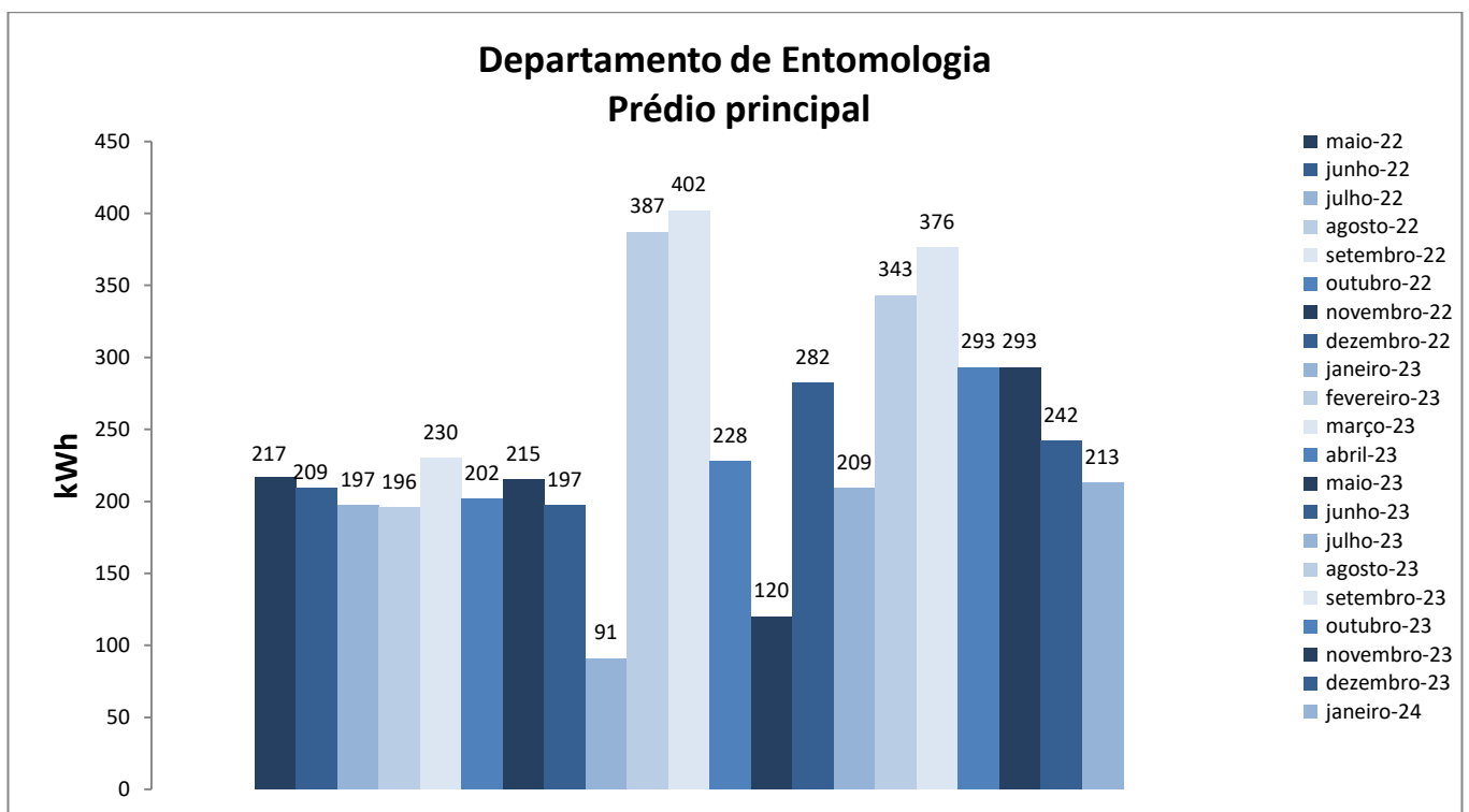
Figura 1. Variação do consumo de energia elétrica da edificação do Departamento de Entomologia
