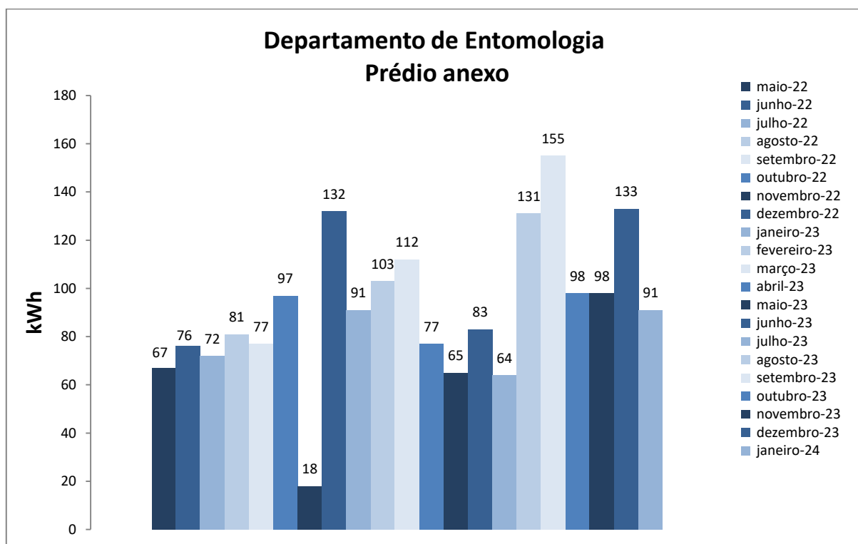
Figura 1. Variação do consumo de energia elétrica da edificação do Departamento de Entomologia - anexo
