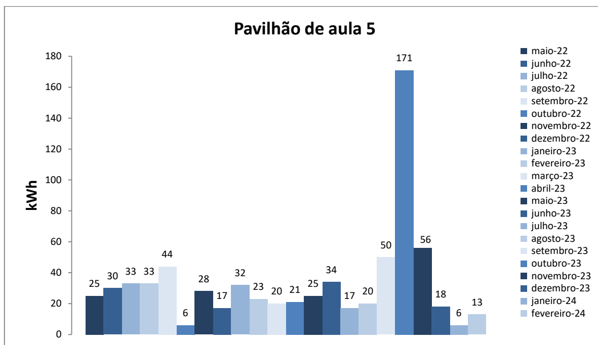
Figura 1. Variação do consumo de energia elétrica da edificação do Pavilhão de Aulas 05.
