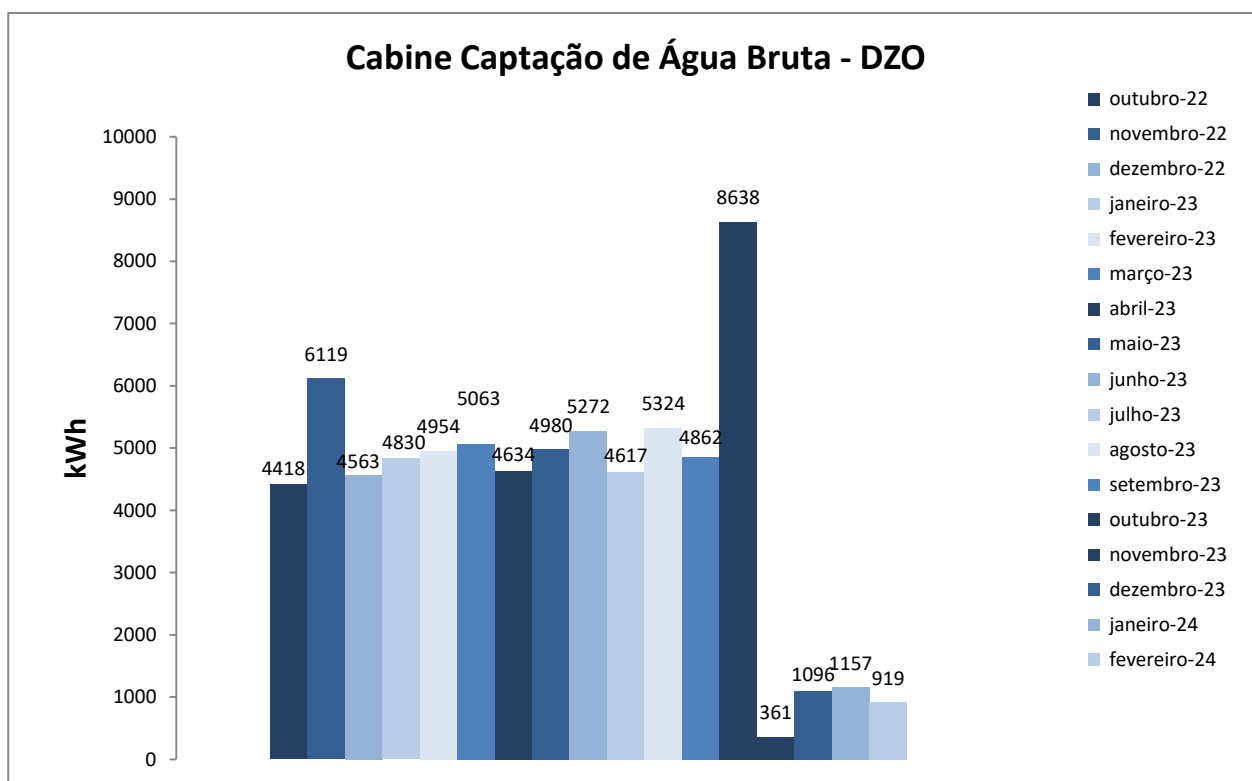
Figura 1. Variação do consumo de energia elétrica da Cabine Barragem Captação Água Bruta - DZO.
