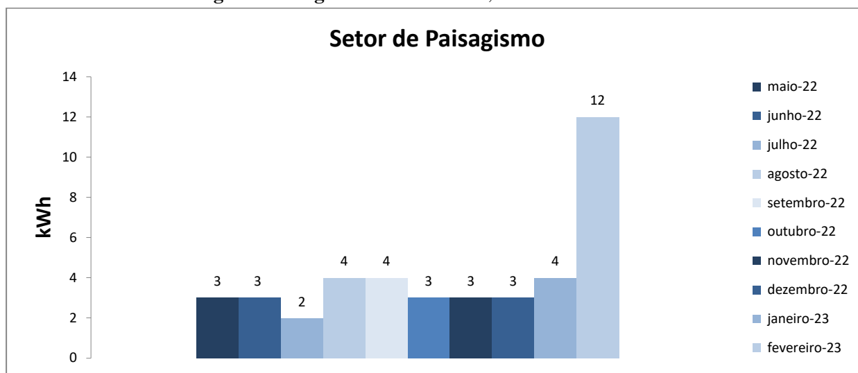
Figura 1. Variação do consumo de energia elétrica da edificação do Setor de Paisagismo.
