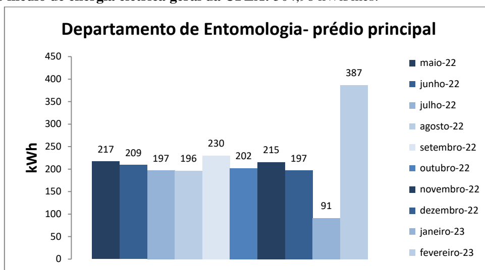
Figura 1. Variação do consumo de energia elétrica da edificação do Departamento de Entomologia Prédio principal
