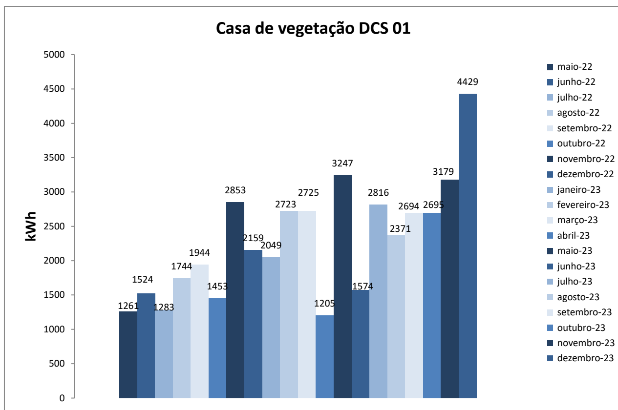
Figura 1. Variação do consumo de energia elétrica da edificação do Departamento de Ciência do Solo Casa de Vegetação 01
