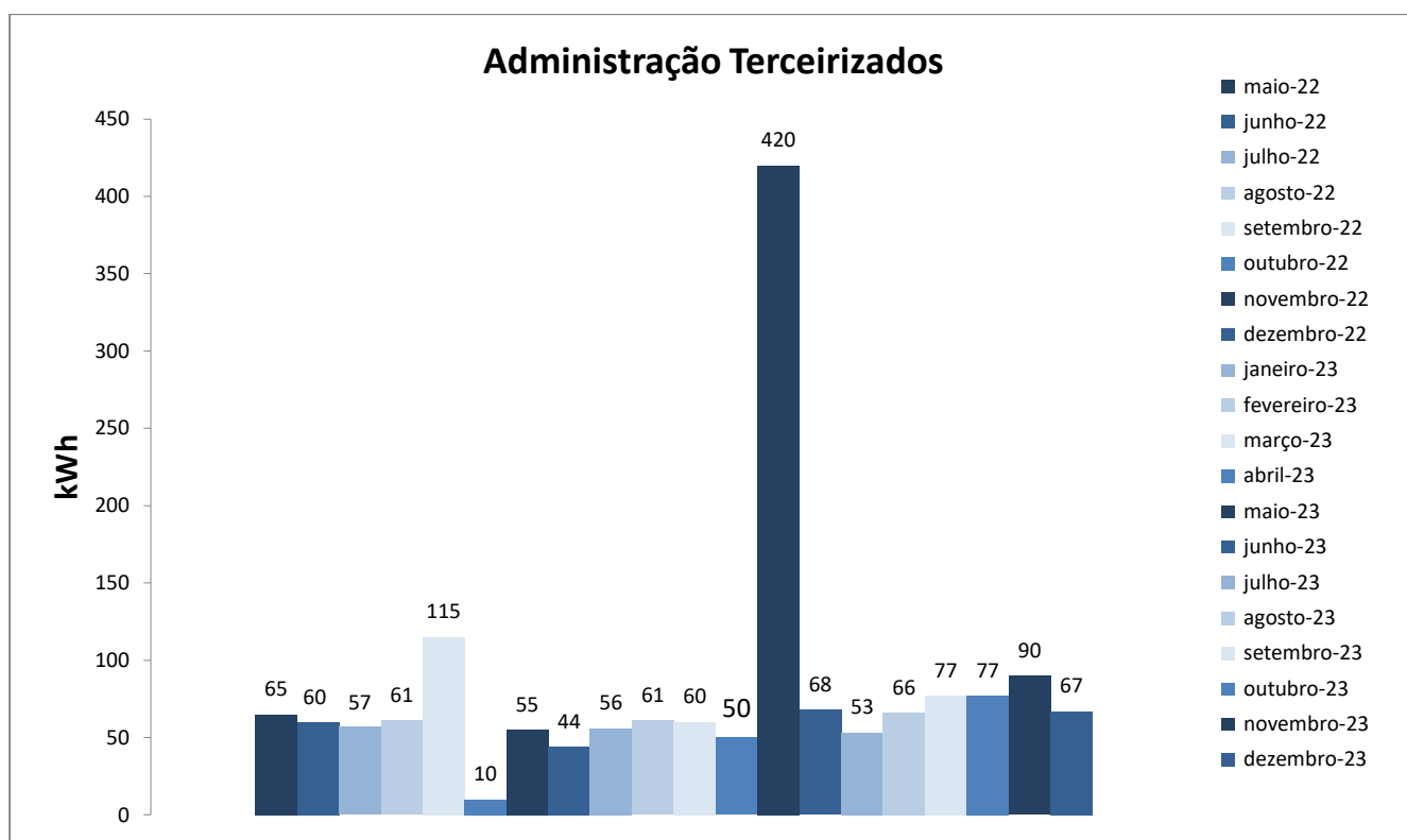
Figura 1. Variação do consumo de energia elétrica do prédio Administrativo Empresas Terceirizadas
