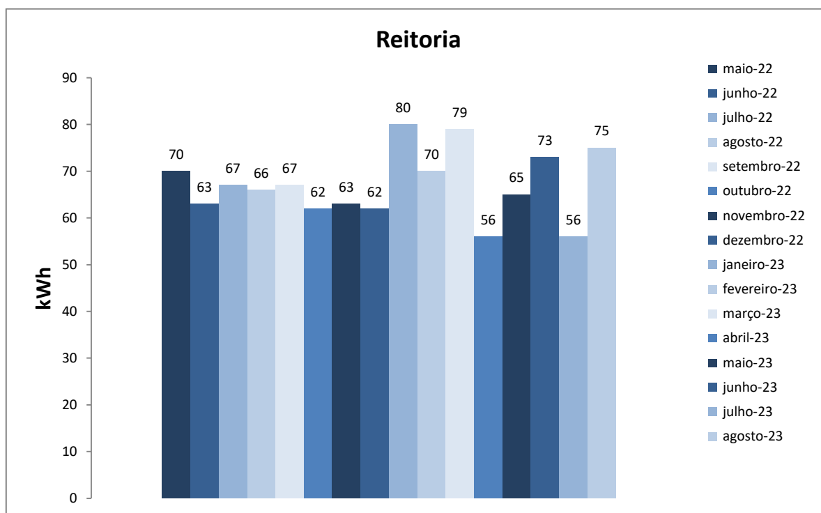
Figura 1. Variação do consumo de energia elétrica da edificação da Reitoria.
