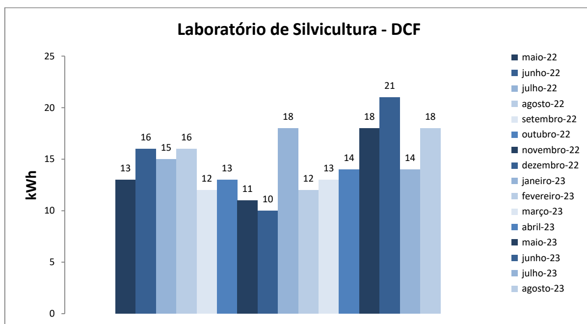
Figura 1. Variação do consumo de energia elétrica da edificação do Laboratório de Silvicultura.
