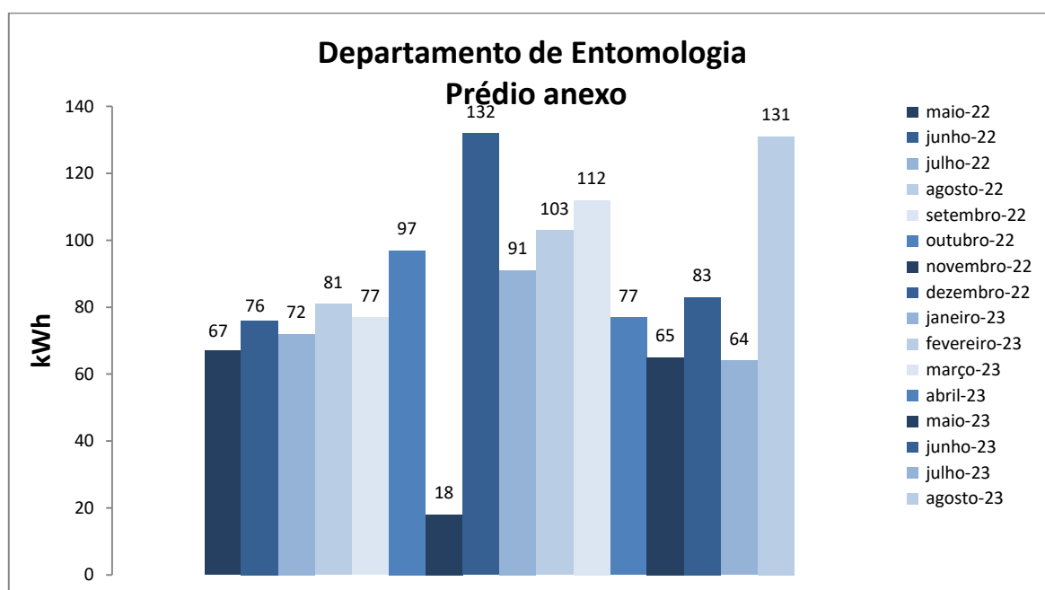
Figura 1. Variação do consumo de energia elétrica da edificação do Departamento de Entomologia - anexo
