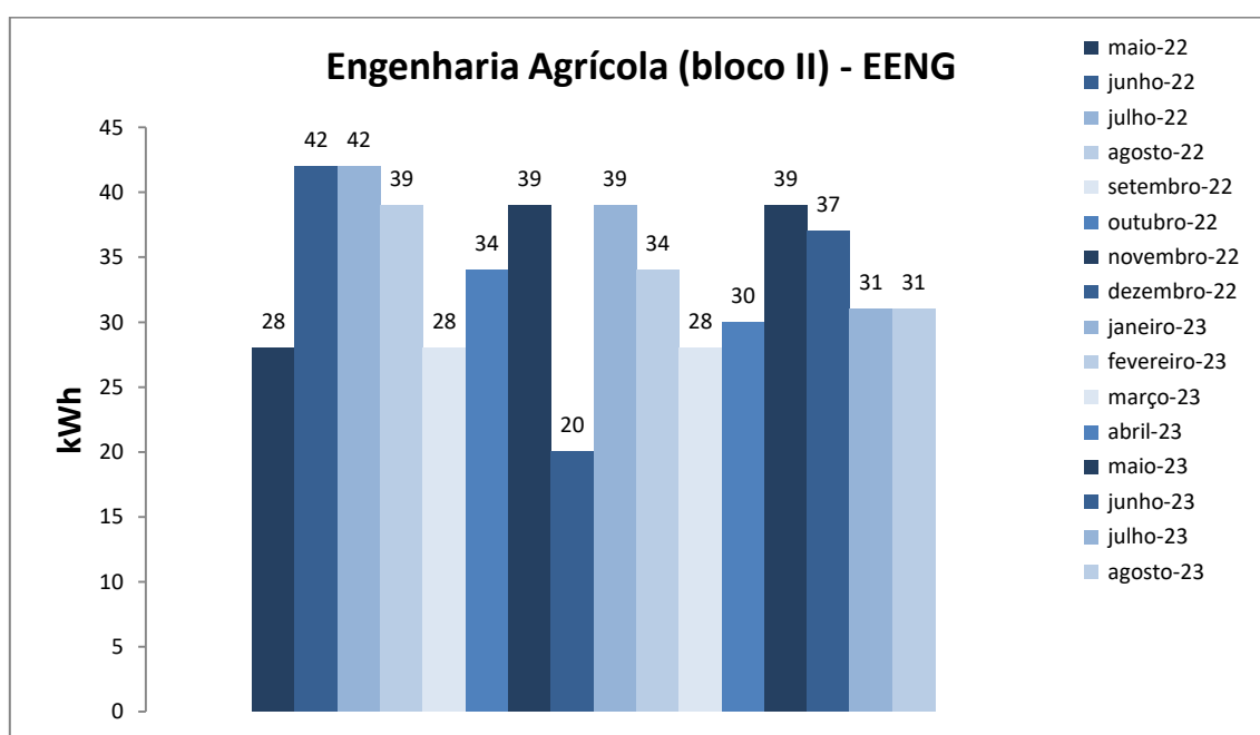
Figura 1. Variação do consumo de energia elétrica da edificação Engenharia Agrícola bloco II.
