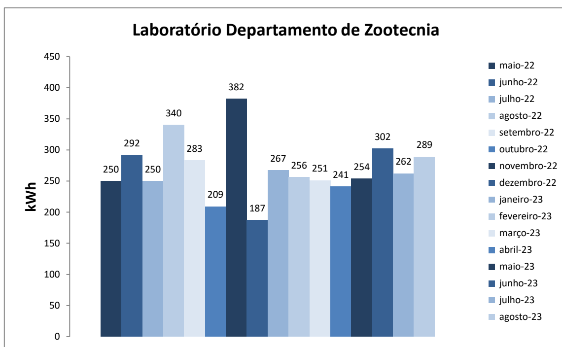
Figura 1. Variação do consumo de energia elétrica da edificação do Laboratório do Departamento de Zootecnia.
