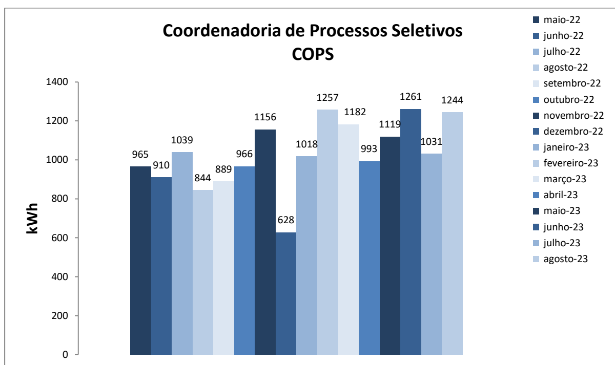
Figura 1. Variação do consumo de energia elétrica da edificação da Coordenadoria de Processos Seletivos
