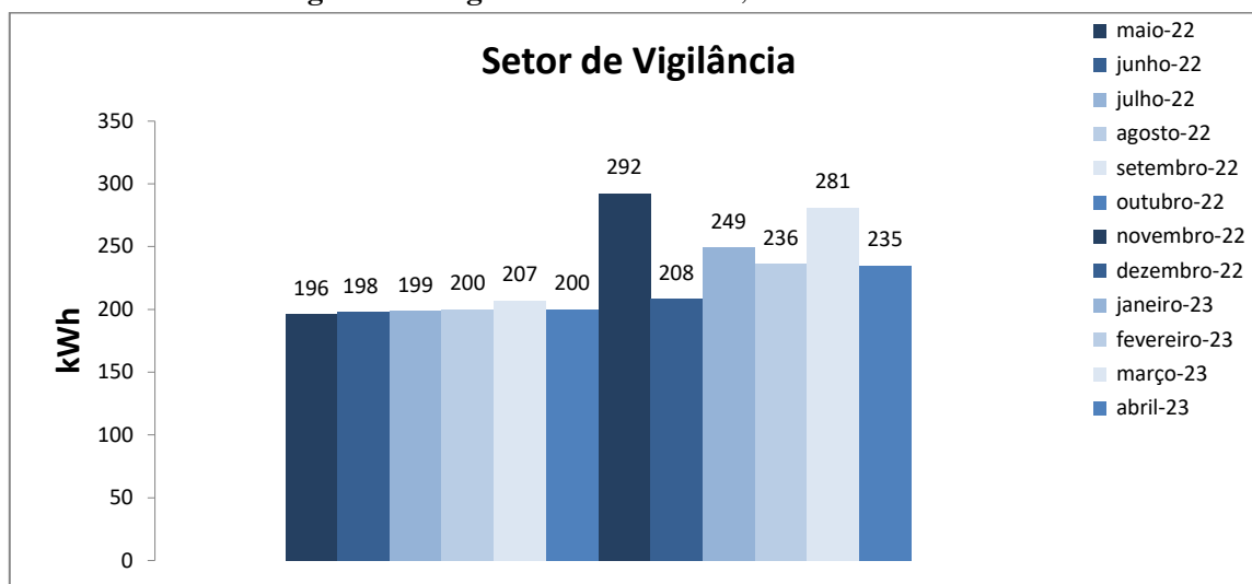
Figura 1. Variação do consumo de energia elétrica da edificação do Setor de Vigilância.
