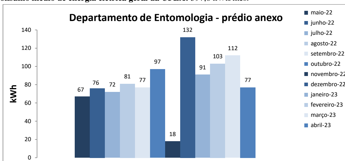
Figura 1. Variação do consumo de energia elétrica da edificação do Departamento de Entomologia-anexo
