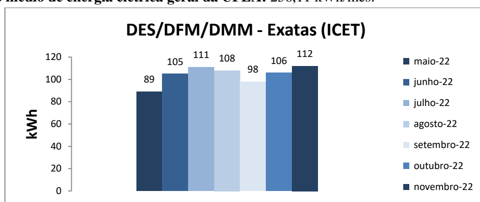
Figura 1. Variação do consumo de energia elétrica da edificação do Departamento de Exatas
