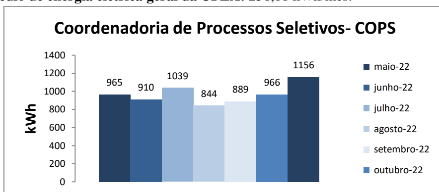
Figura 1. Variação do consumo de energia elétrica da edificação da Coordenadoria de Processos Seletivos - COPS.
