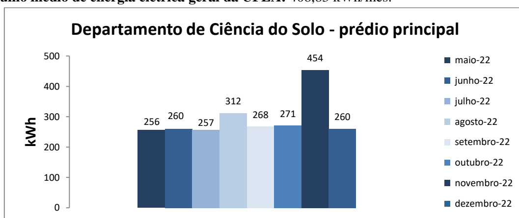
Figura 1. Variação do consumo de energia elétrica da edificação do Departamento de Ciência do Solo Prédio principal
